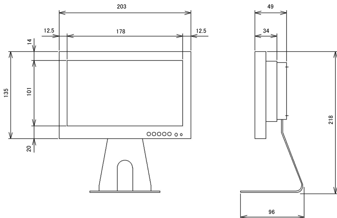
外形寸法図／NM-LCDWB80M
