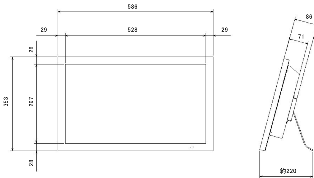
外形寸法図／NM-LCDW238-HDR
