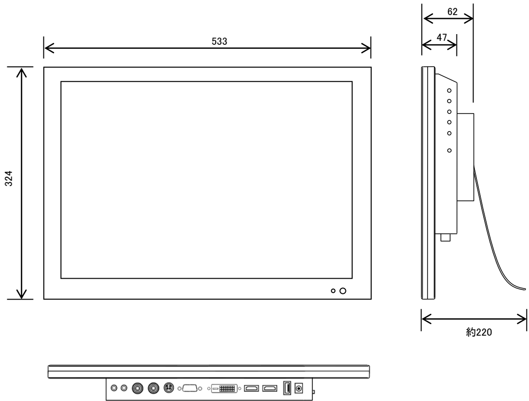
外形寸法図/NM-LCDW215HME
