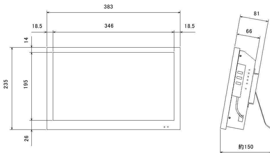
外形寸法図／NM-LCDW156CPU
