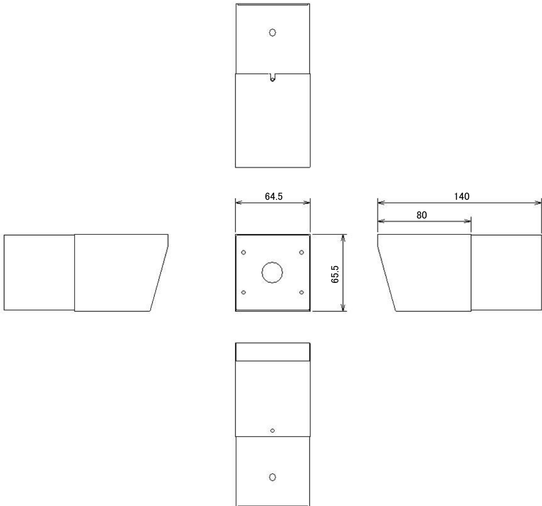
外形寸法図／NM-J110-V
